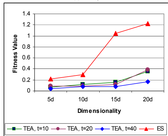
(b) Griewank
