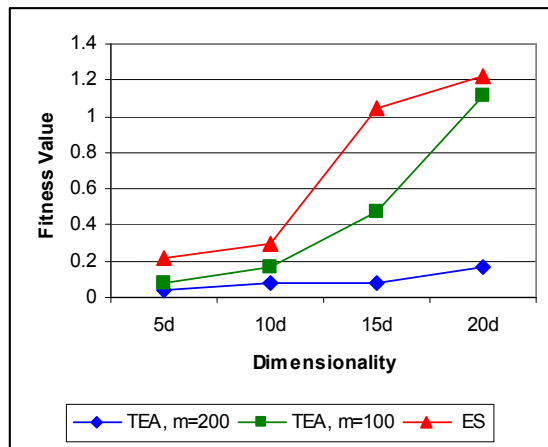
(b) Griewank
